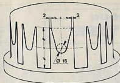
Allègement de l'embrayage
