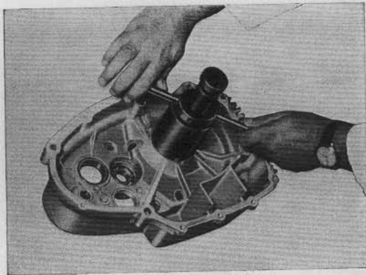
24 - Estrattore per cuscinetti 88713.0269
