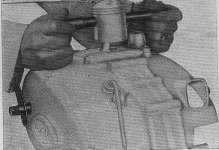
16-17 - Spina per montaggio e smontaggio spinotto pistone 88713.0450/0431
