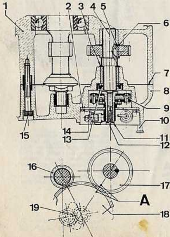
Coupe de la pompe à huile à engrenages : 1. Orifice de refoulement de l'huile - 2 et 3. Ressort et bille de tarage - 4. Corps de pompe - 5. Arbre de la pompe avec son embout d'accouplement du type à tenon - 6. Fil de fer de sécurité pour interdire le desserrage des vis - 7. Vis d'assemblage du corps de pompe sur le couvercle arrière droit - 8. Rondelle-frein - 9. Flasque intérieure de la pompe - 10. Joint - 11. Orifice d'admission de l'huile - 12. Couvercle arrière droit du carter-moteur
