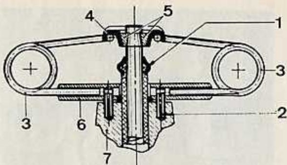
Montage des ressorts épingle (3) de rappel d'une soupape
