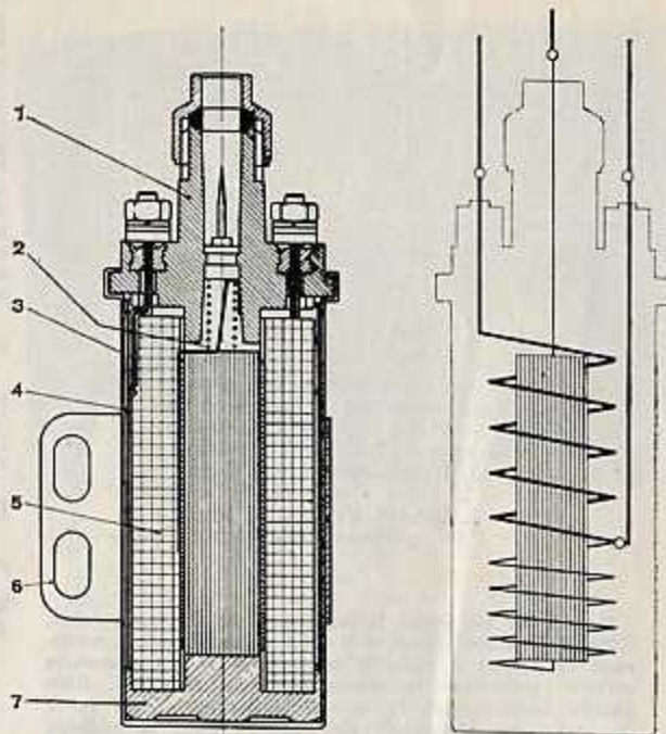
Bobine H.T. d'allumage : 1. Couvercle - 2. Ressort - 3. Boîtier - 4. Protection anti-magnétique - 5. Enroulement primaire et secondaire - 6. Support - 7. Fond protecteur
