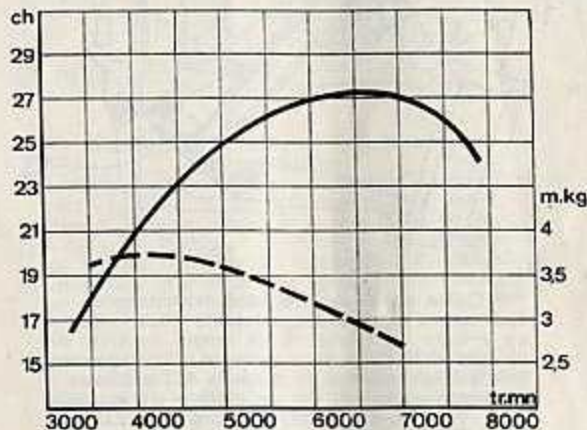
Courbes de puissance et de couple du 450
