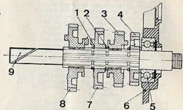
Arbre secondaire et pignons de la boîte de vitesses : 1 et 2. Rondelles et circlips - 8, 7, 3 et 4. Pignons de 2 e , 3 e , 4 e et 5 e vitesse de l'arbre secondaire - 5. Roulement à billes - 6. Carter-moteur - 9. Arbre secondaire
