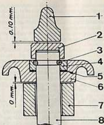
Position des pièces de la distribution desmodromique
