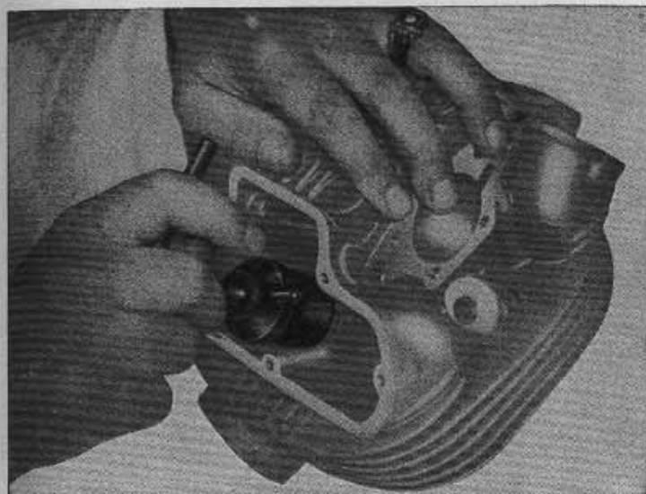
8 - Pinza per smerigliare sedi valvole 88713.0257
