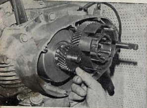
L'extraction du petit pignon de transmission primaire ne pose pas de problème du fait de son emmanchement droit avec clavette sur le vilebrequin (photo R.M.T.)
