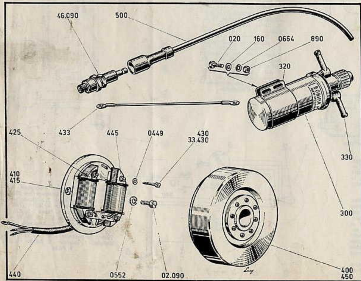
Equipement électrique à volant magnétique
