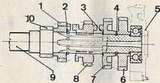
Arbre primaire et pignons de la boîte de vitesses 10, 1, 8, 7 et 6. Pignons de 1 er , 2 e , 3 e , 4 e et 5 e vitesse de l'arbre primaire - 2. Rondelle et circlip - 3. Rondelle - 4. Circlip - 5. Carter-moteur - 9. Arbre primaire avec son pignon usiné (10) de première vitesse
