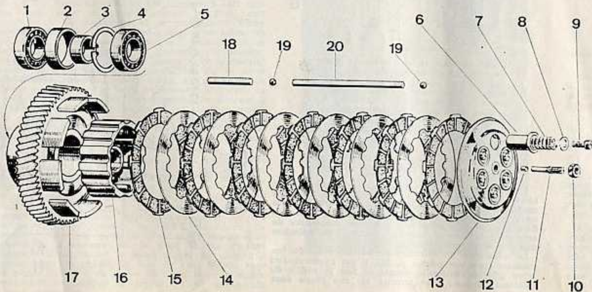
Embrayage multidisque du type à bain d'huile : 1 et 5. Deux roulements 20 × 42 × 08 - 2. Entroise extérieure - 3. Entroise intérieure - 4. Circlip de calage - 6. Guides des ressorts - 7. Ressorts hélicoïdaux - 8 et 9. Rondelle et vis de compression des ressorts - 10 et 11. Contre-écrou et vis de réglage de la butée d'embrayage - 12. Galet de la commande d'embrayage - 13. Plateau de pression - 14. Disques lisses - 15. Disques garnis - 16. Noix d'embrayage - 17. Cloche d'embrayage venant de fonderie avec le pignon de transmission primaire - 18, 19 et 20. Tiges et billes de commande d'embrayage traversant l'arbre primaire de la boîte de vitesses
