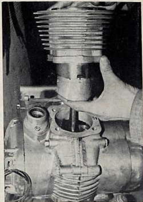
Après avoir parfaitement rentré les segments dans leur gorge, le poids du cylindre doit suffire pour provoquer sa descente. Il ne faut surtout pas forcer au risque de casser un segment (photo R.M.T.)
