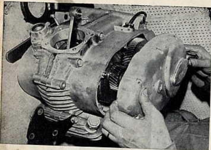
La dépose du couvercle d'embrayage permet l'accessibilité à l'embrayage, à la transmission primaire, au kick-starter (1 er modèle) et à l'alternateur (ou au volant magnétique) (photo R.M.T.)
