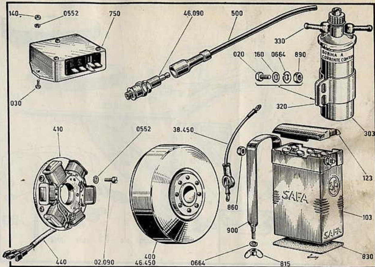
Equipement électrique avec alternateur à 6 bobinages : 400. Rotor de l'alternateur - 410. Stator de l'alternateur - 750. Bloc redresseur régulateur de courant
