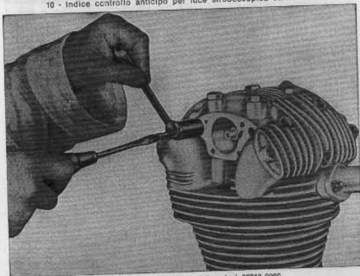
11 - Estrattore per perno bilancieri 88713-0260 Estrattore per perno bilancieri DESMO 88713-0435
