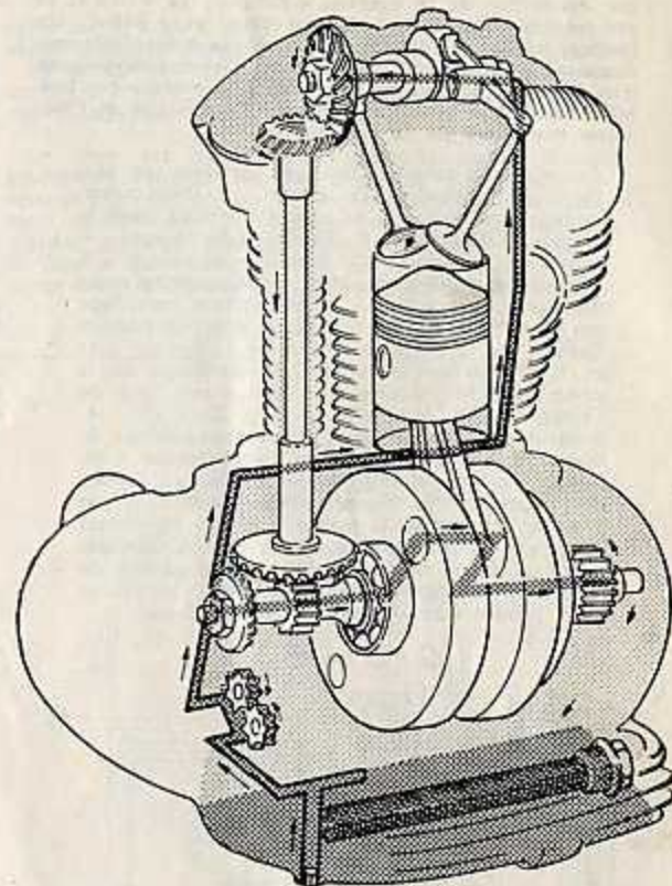
Circuit de graissage des monocylindres Ducati
