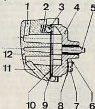
Coupe de la pompe à huile à engrenages : 1. Orifice de refoulement de l'huile - 2 et 3. Ressort et bille de tarage - 4. Corps de pompe - 5. Arbre de la pompe avec son embout d'accouplement du type à tenon - 6. Fil de fer de sécurité pour interdire le desserrage des vis - 7. Vis d'assemblage du corps de pompe sur le couvercle arrière droit - 8. Rondelle-frein - 9. Flasque intérieure de la pompe - 10. Joint - 11. Orifice d'admission de l'huile - 12. Couvercle arrière droit du carter-moteur
