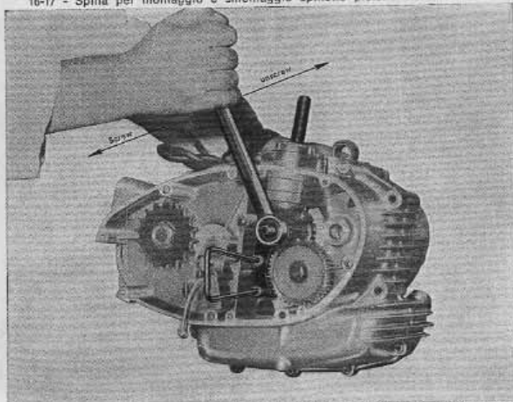
18 - Attrezzi fissa-albero motore per bloccare ingranaggio conico Z = 21 88713.0266 screw - svitare unscrew - svitare
