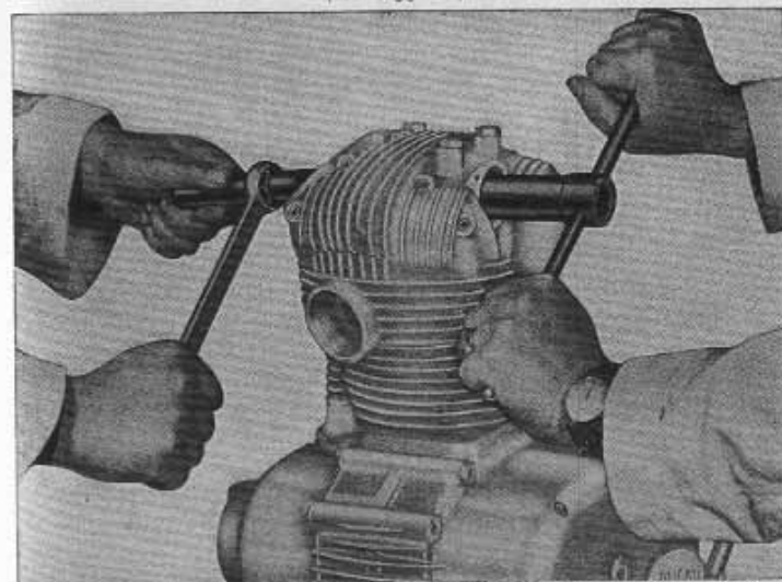
15 - Chiave fissa-albero distribuzione per bloccare ingranaggio conico Z=28 88713-0263
